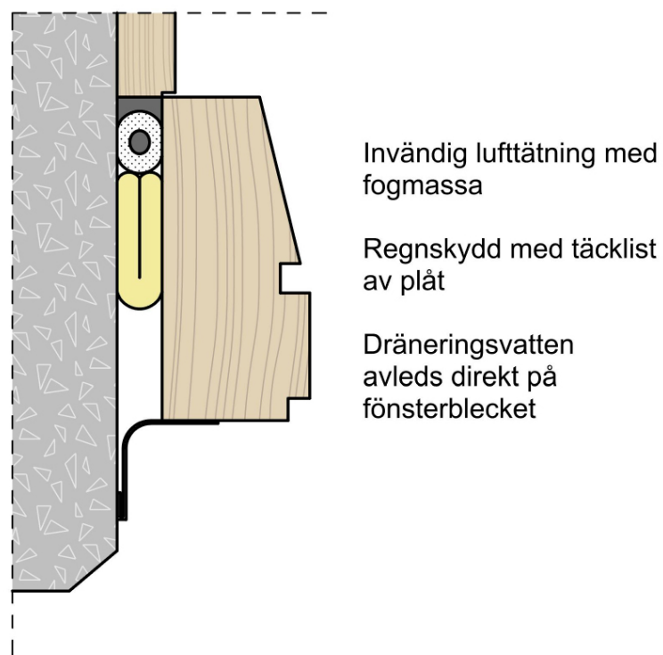
FIGUR 4A. Fog mellan karmsidostycke av trä och lättbetongvägg
