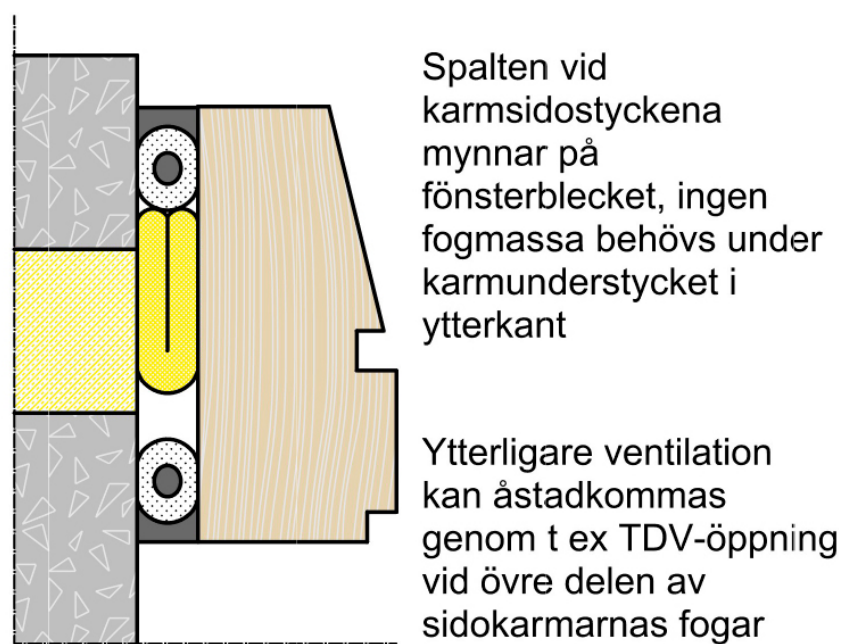
FIGUR 3A. Fog mellan karmsidostycke av trä och betongelement
