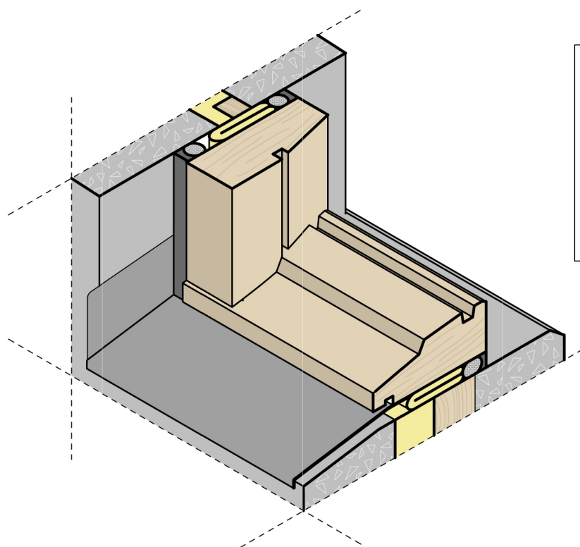
FIGUR 3B. Fog mellan karmsidostycke av trä och betongelement TDV-öppning övre delen av sidokarmarnas fogar.
