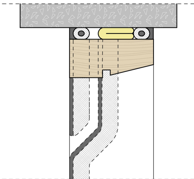
FIGUR 3B. Fog mellan karmsidostycke av trä och betongelement TDV-öppning övre delen av sidokarmarnas fogar.
