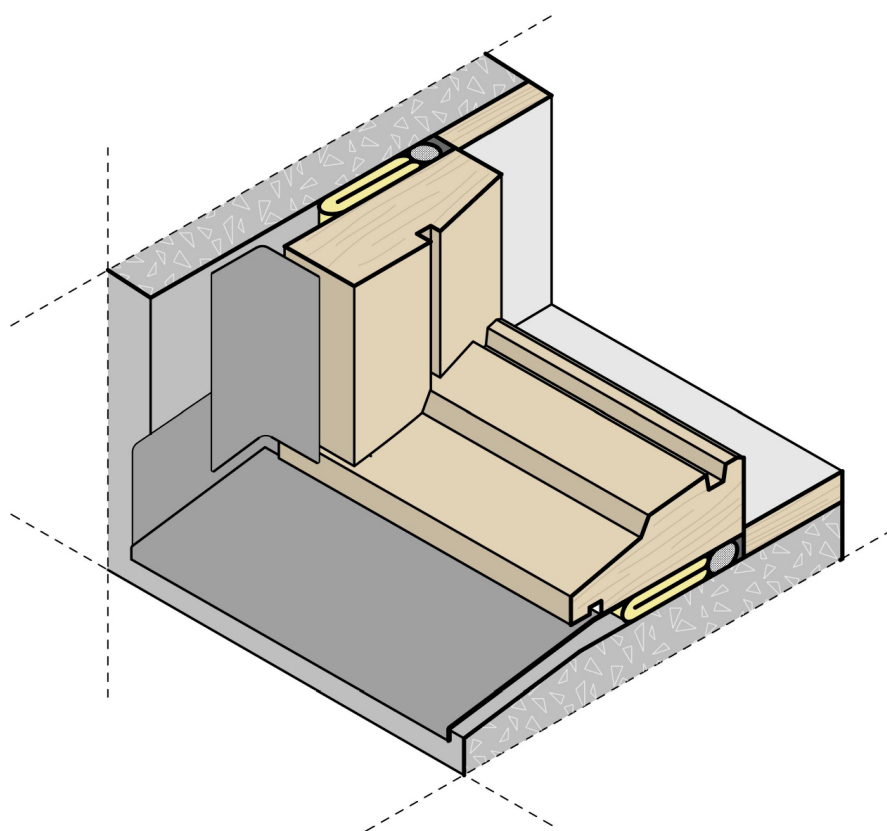
FIGUR 4B. Fog mellan karmsidostycke av trä och lättbetongvägg
