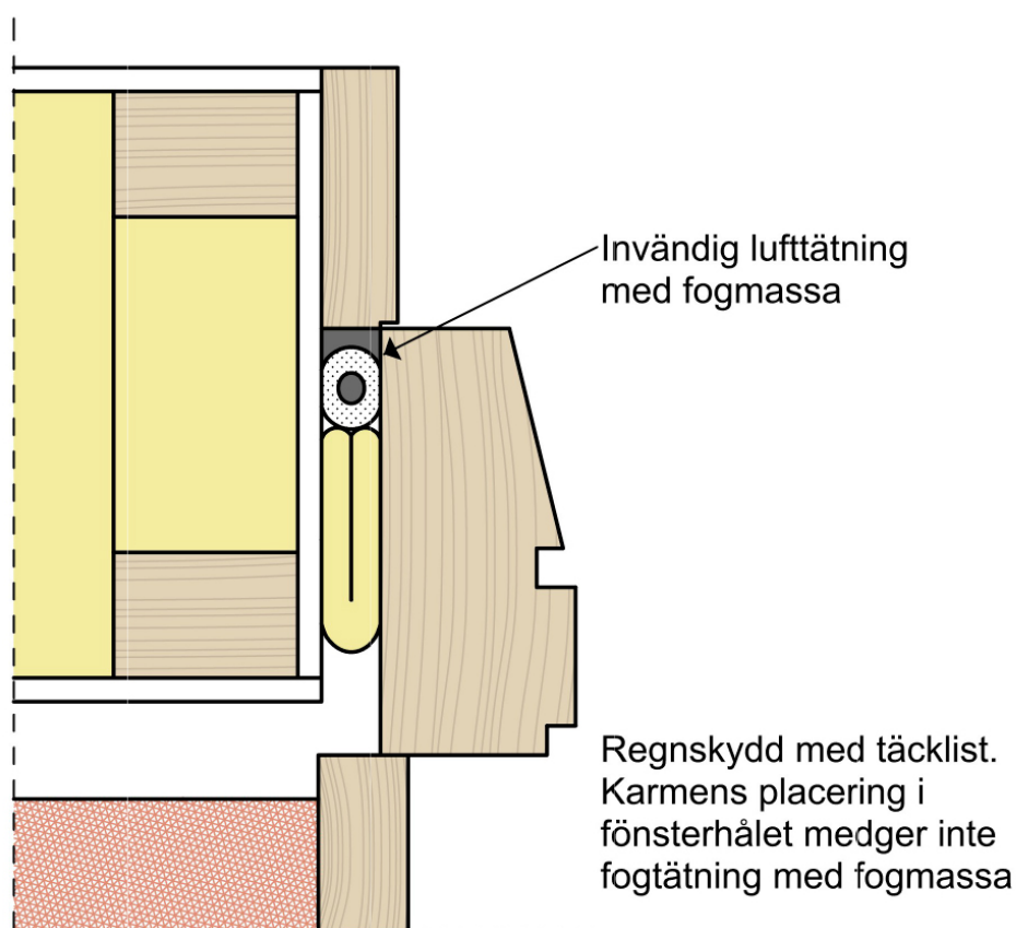
FIGUR 2A. Fog mellan fönsterkarm av trä och träregelvägg med skalmur
