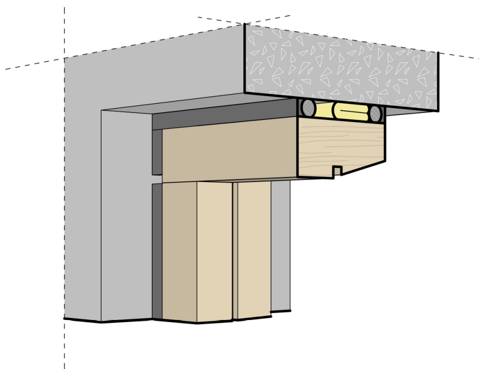
FIGUR 5A. Fönsterkarm, övre vänstra hörn. Ventilerings genom TDV-lösning kan med fördel göras med överlappande fog.
