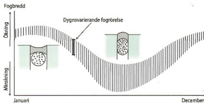
Figur 2. Schematisk bild av årtids- och dygnsvarierande fogrörelser under ett år i en yttervägg. På vintern ökar fogbredden och på sommaren minskar den [3].
