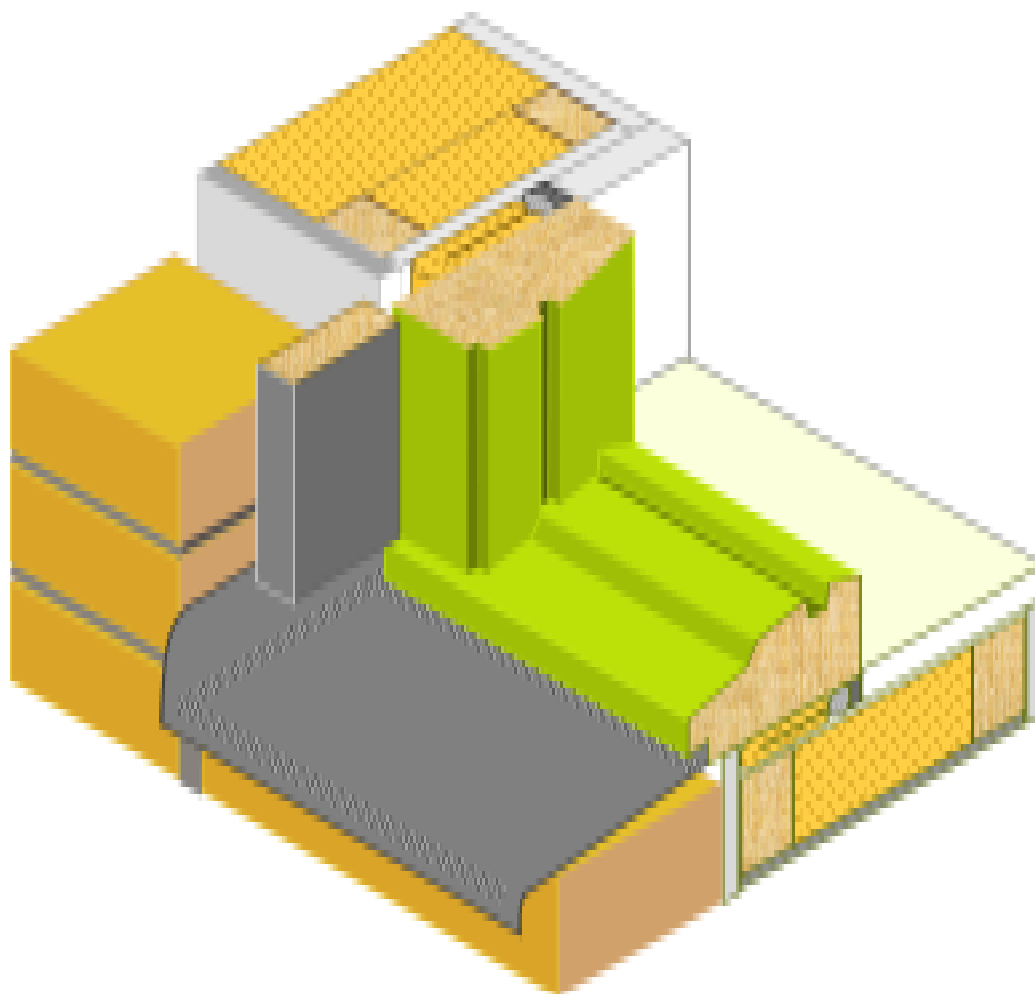
FIGUR 2. Fog mellan fönsterkarm av trä och träregelvägg med skalmur
