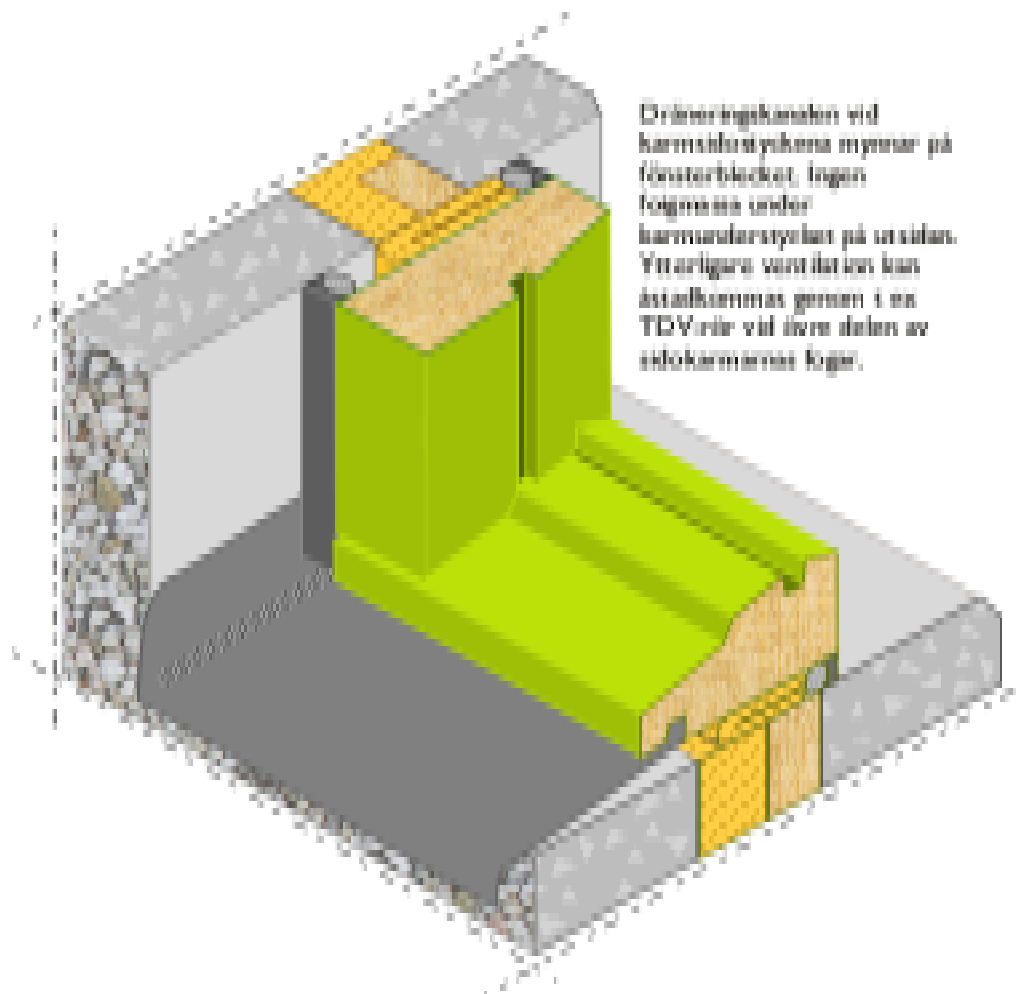
FIGUR 3. Fog mellan karmsidostycke av trä och betongelement
