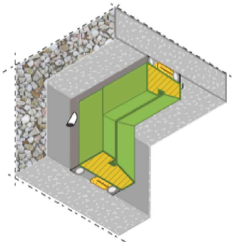
FIGUR 5A. Fönsterkarm, övre vänstra hörn. Ventilering genom TDV-lösning kan med fördel göras med överlappande fog.
