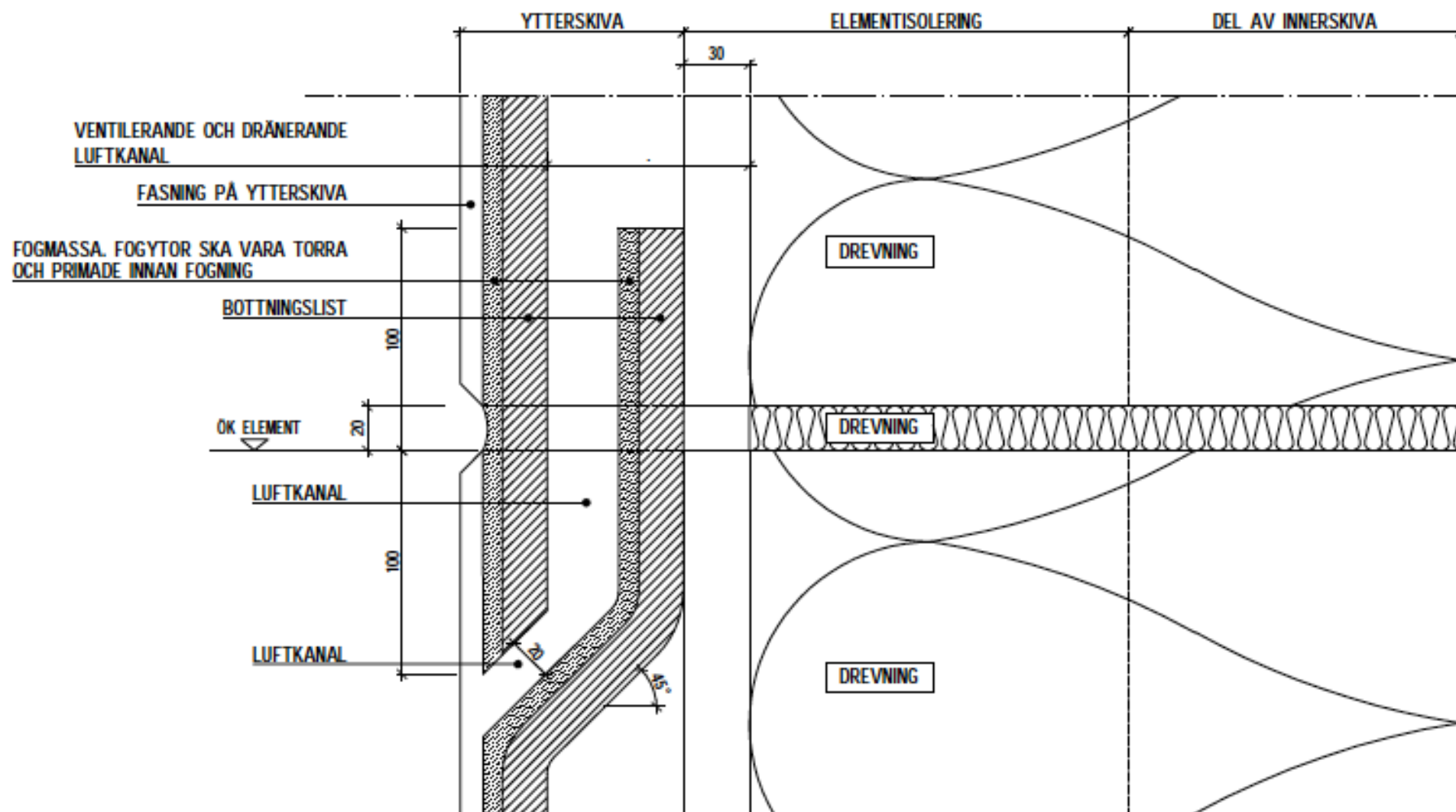
B- PRINCIPDETALJ VERTIKALA FOGAR I PREFAB YTTERVÄGG 1:2 VERTIKALSNITT.
