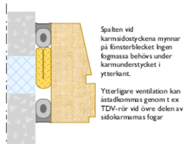
FIGUR 2. Fog mellan fönsterkarm av trä och träregelvägg med skalmur
